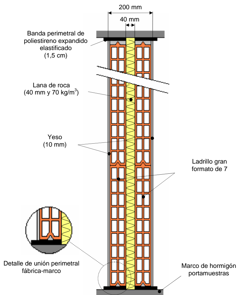
Figura 1: Esquema de la muestra ensayada (B0141-04-M241)
