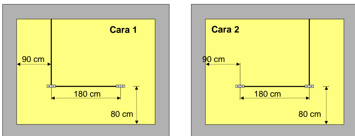
Figura 3: Ubicación de las rozas en ambas caras de la muestra
