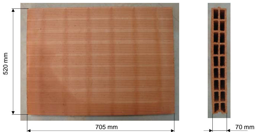
Figura 2: Dimensiones medidas del ladrillo gran formato de 7
