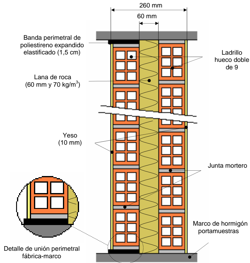
Figura 1: Esquema de la muestra ensayada (B0103-06-M124)
