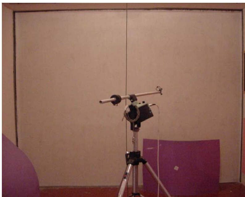
Foto 4: Vista de la muestra en cámaras de ensayo
